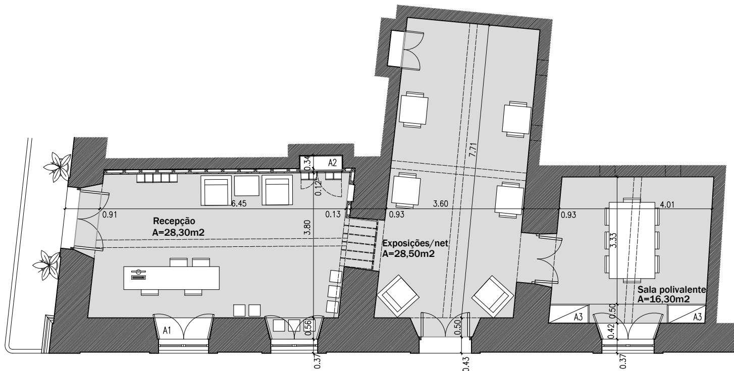
Planta Geral
