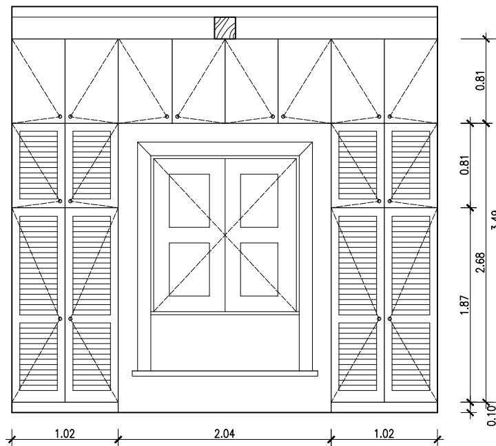
ALÇADO EXTERIOR
